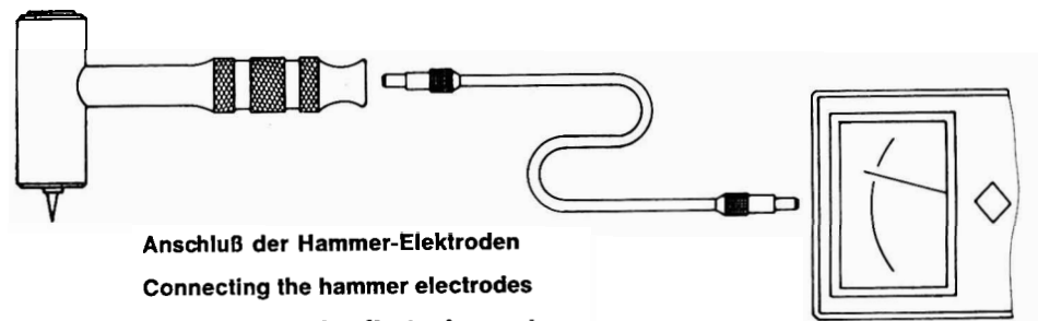
Raccordement des électrodes-marteaux
